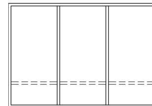
AANZICHT ZIJWAND MET OPTIONEEL HORIZONTALE TUSSENREGEL
